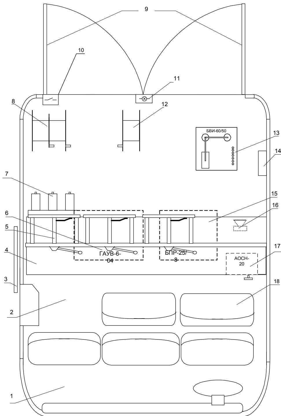
Рис.1. Схема размещения оборудования лаборатории КАЭЛ-3 в фургоне автомобиля
