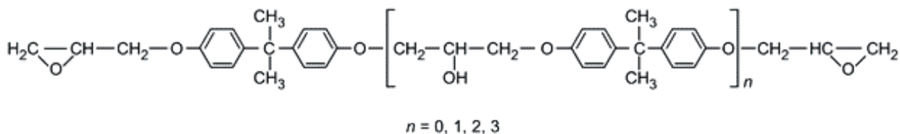
Рисунок А.1 - Молекулярная структура эпоксидной смолы
