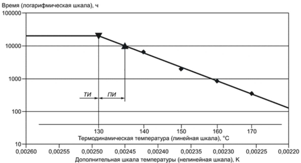
Рисунок А.2 - График теплостойкости
